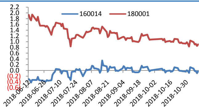
图1 主力TF 合约活跃CTD基差走势
