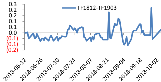
图2 TF 合约跨期价差
