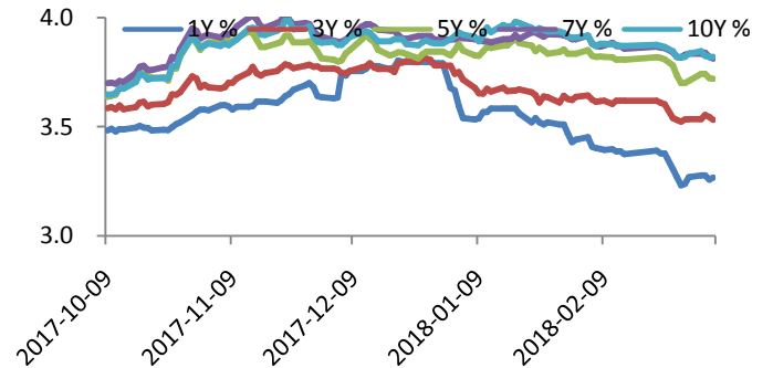
图10 银行间国债 YTM 走势
