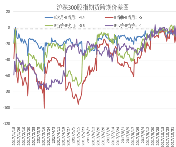
图 3.4 沪深 300 股指期货跨期价差图
