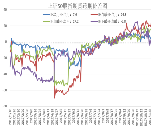
图 3.5 上证 50 股指期货跨期价差图
