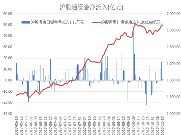
图 1.1 沪股通资金净流入(亿元)
