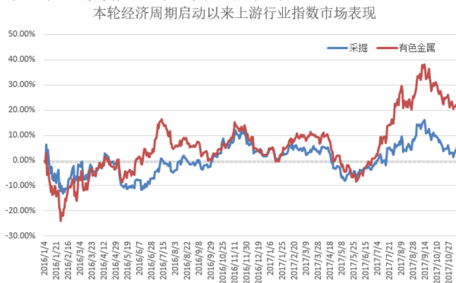
图 4.1 本轮经济周期启动以来上游行业指数市场表现
