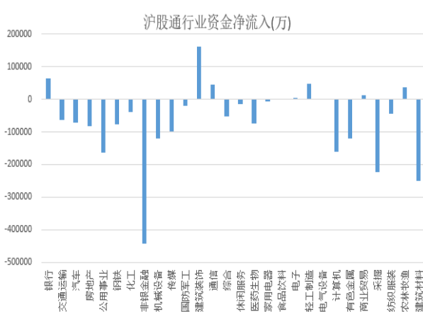
图 1.3 沪股通行业资金净流入
