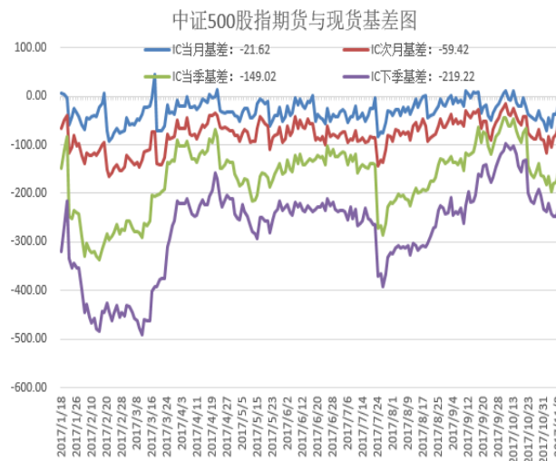
图 3.3 中证 500 股指期货与现货基差图
