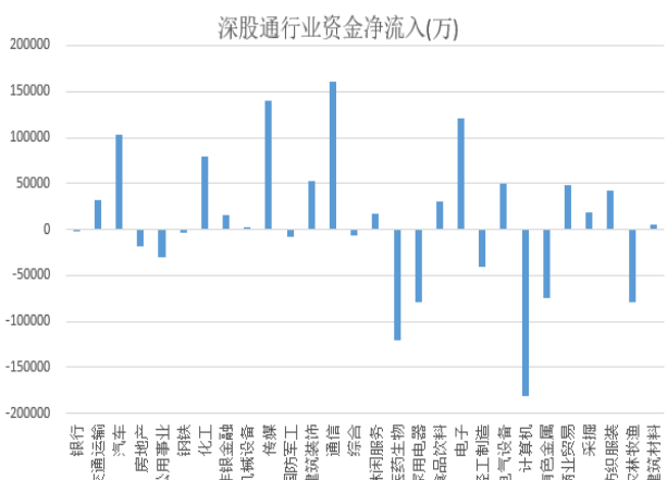
图 1.4：深股通行业资金净流入
