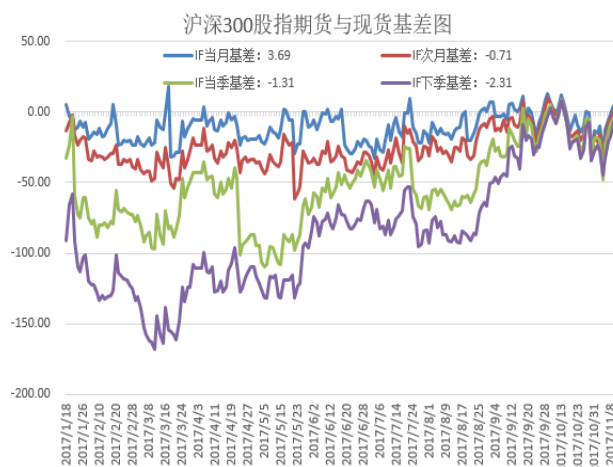
图 3.1 沪深 300 股指期货与现货基差图
