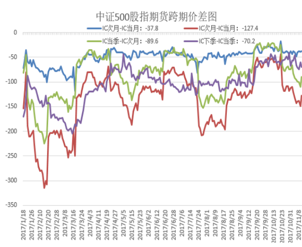
图 3.6 中证 500 股指期货跨期价差图
