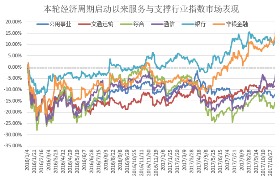
图 4.4 本轮经济周期启动以来服务与支撑行业指数市场表现
