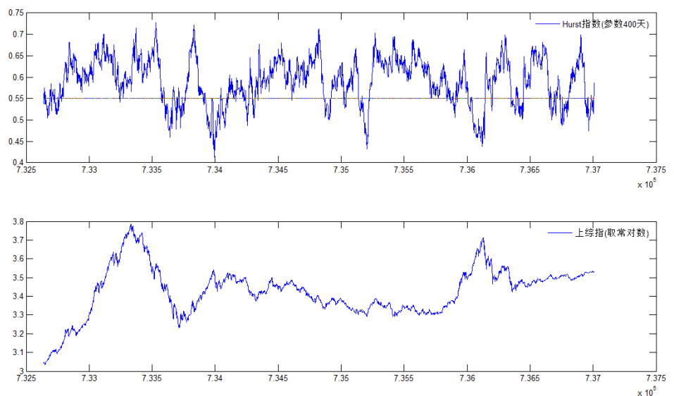
图 5.1 上证综指与 Hurst 指数(截止 2017-11-10)
