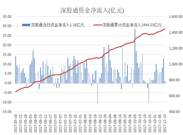
图 1.2：深股通资金净流入(亿元)
