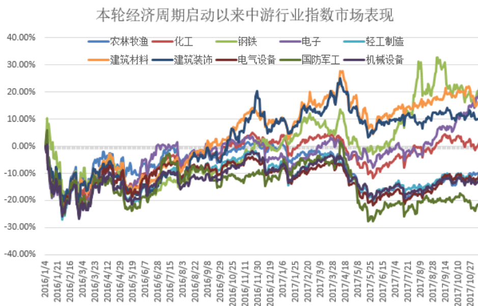
图 4.2 本轮经济周期启动以来中游行业指数市场表现
