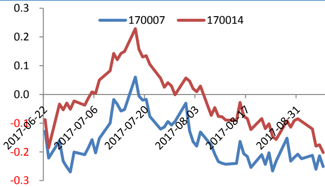
图1 主力TF 合约活跃 CTD 基差走势
