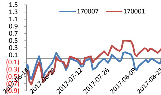
图 1 主力 TF 合约活跃 CTD 基差走势
