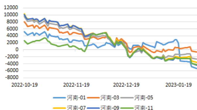
基差走势图
